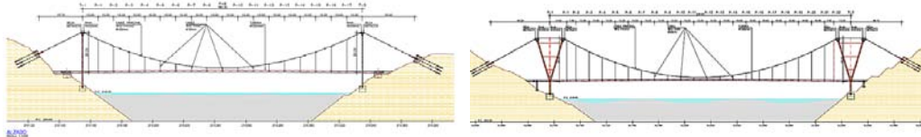
Figura 14. Estructuras de paso de la tubería de abastecimiento Portaje-Cáceres sobre el Almonte (180 m de vano) y sobre el Tajo (230 m de vano), en fase de proyecto. La cercanía a los puentes de la A-66 puede convertir en un desastre paisajístico la oportunidad existente de poder disfrutar de cuatro estructuras singulares en un mismo entorno.
